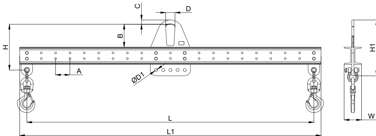
タイプA 1点吊り用
