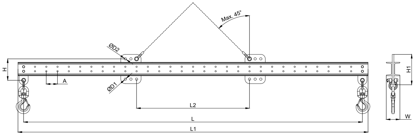
タイプB 2点吊り用
